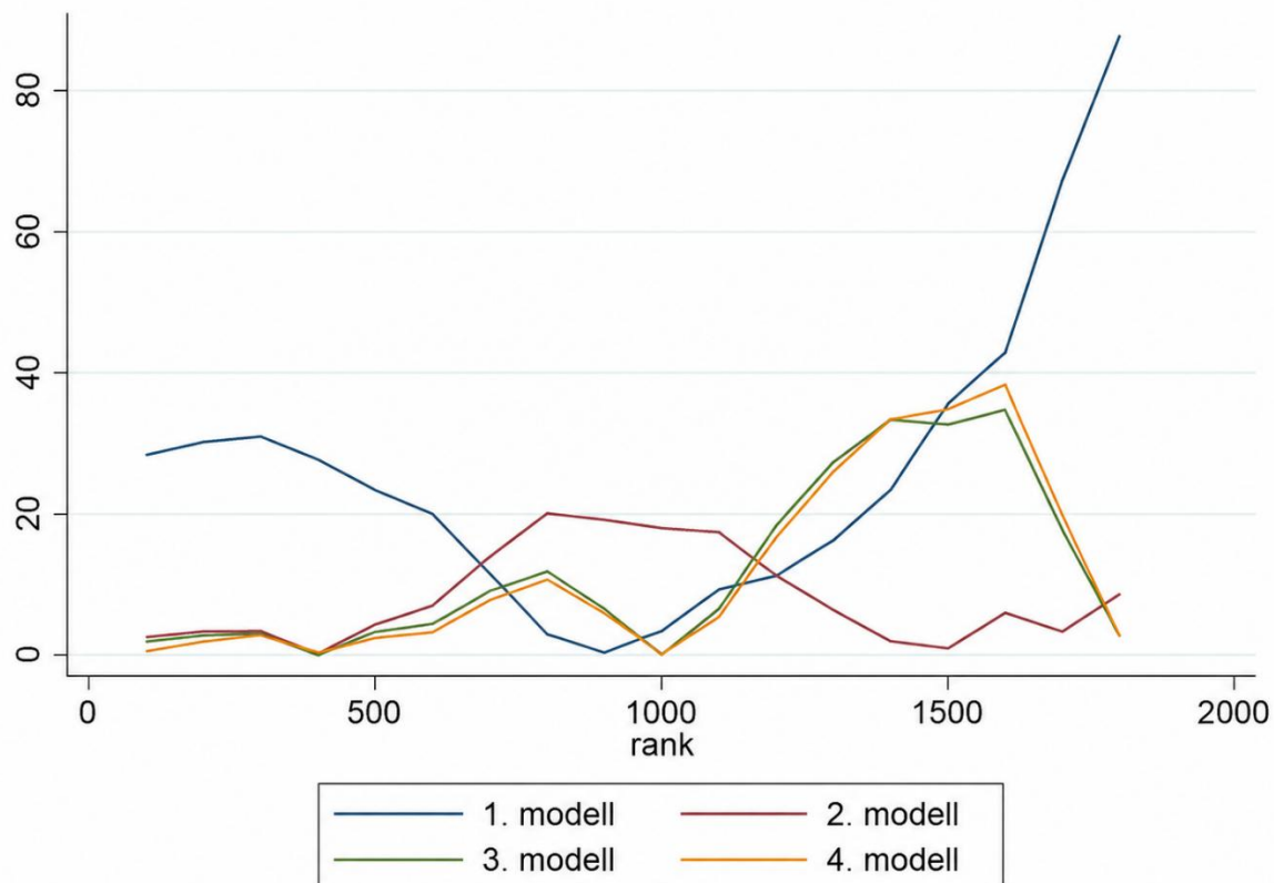
6. ábra: Abszolút predikciós hiba S görbe és ötödrendű polinom
