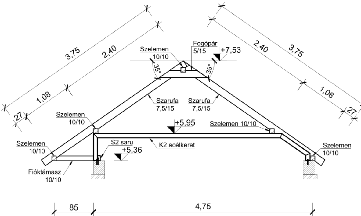
Fedélszék B-B metszet
