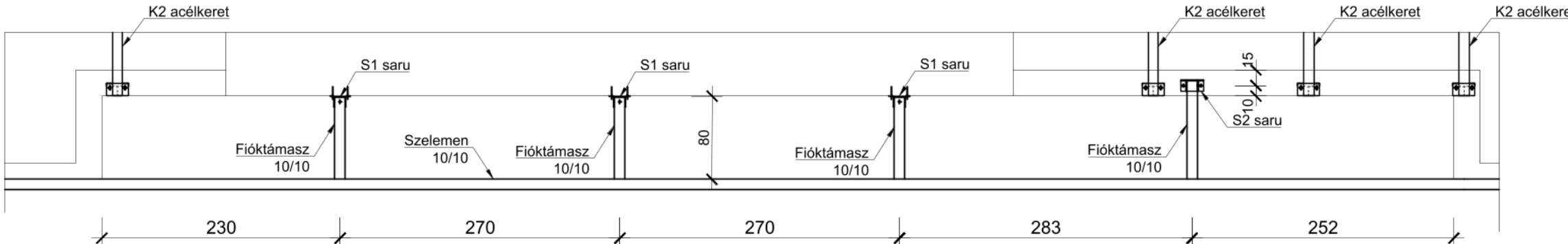
Fedélszék D-D metszet
