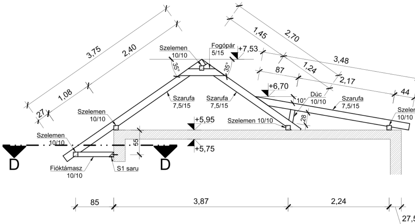
Fedélszék A-A metszet
