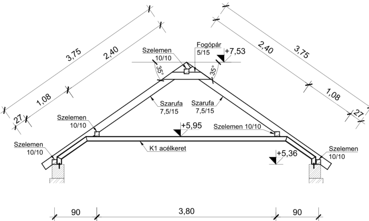
Fedélszék C-C metszet
