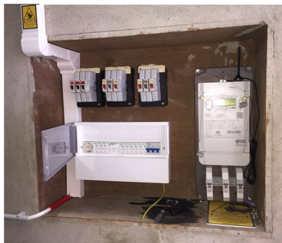
A lakáselosztó faliszekrény
