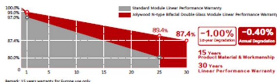
Linear map
