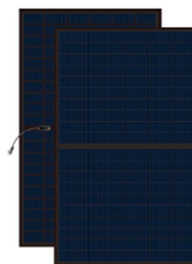
Module diagram
