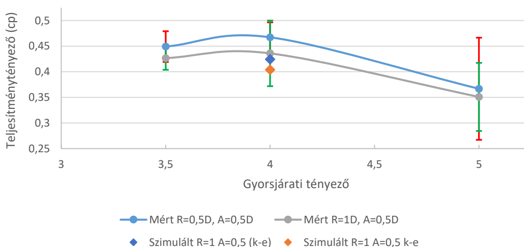
79. ábra. R = 0,5D, A = 0,5D és R = 1D, A = 0,5D konfigurációjú ikerturbinák mért és szimulált teljesítménytényezői \lambda = 4 gyorsjárat tényező esetén, tranziens szimuláció, k - \epsilon turbulenciamodellel
