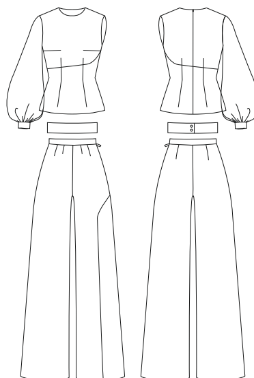
4.2. ábra Bori- modell gyártmányrajz
