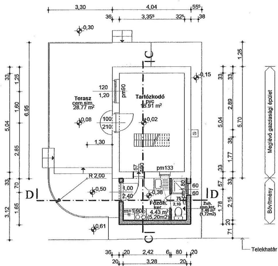
2.22. ábra: A földszinti alaprajz
