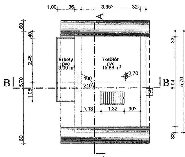
2.23. ábra: A tetőtér alaprajza
