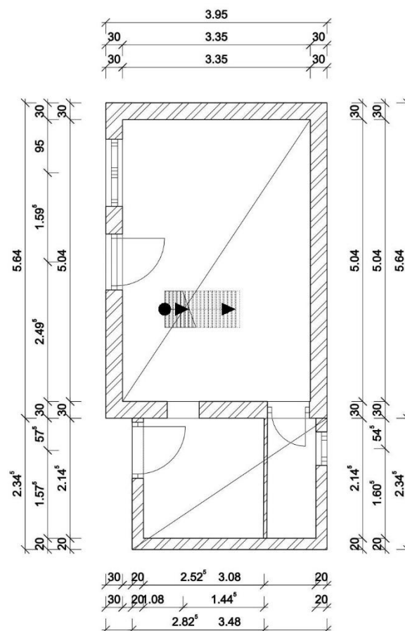
3.1. ábra: Alaprajz az új ajtónyílással
