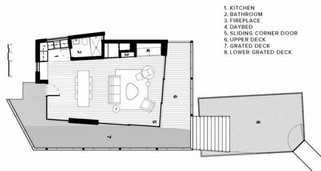
2.8. ábra: Az alaprajz
