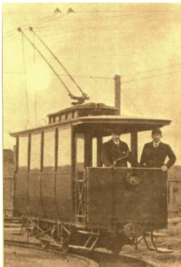
3. kép: 500 V-os kétfázisú próbakocsi a Ganz próbapályán, 1896.
