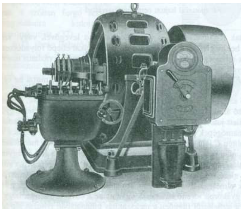
2. kép: Nagyteljesítményű „FF” jelű indukciós motor
