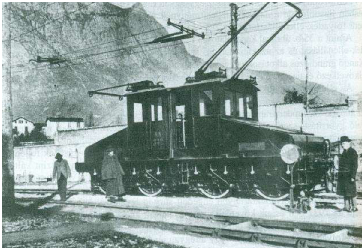
6. kép: Az RA 34 sorozatú háromfázisú mozdony
