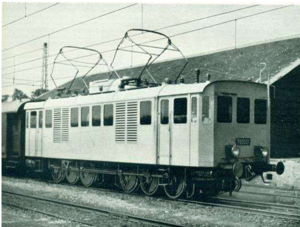
20. kép: A V60-as sorozatú fázisváltós mozdony
