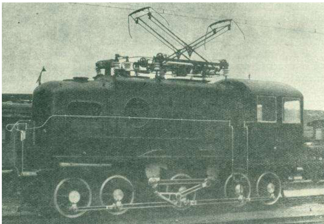
14. kép: Az első fázisváltós próbamozdony, 1923.
