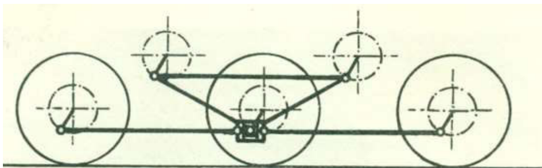
8. kép: A Kandó-keret, vagy Kandó-háromszög vázlata
